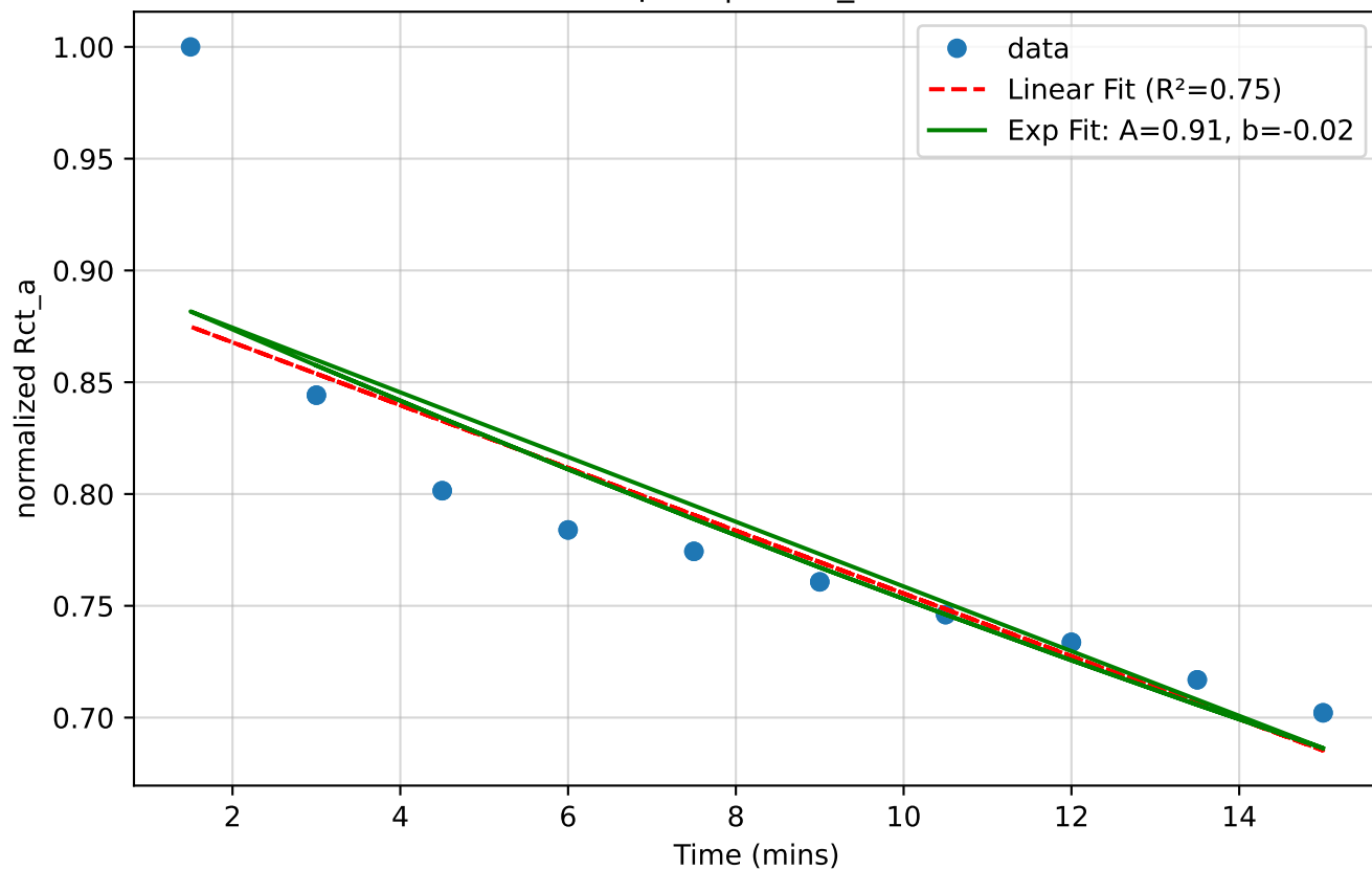
Chip 39 | 10nM_asso
