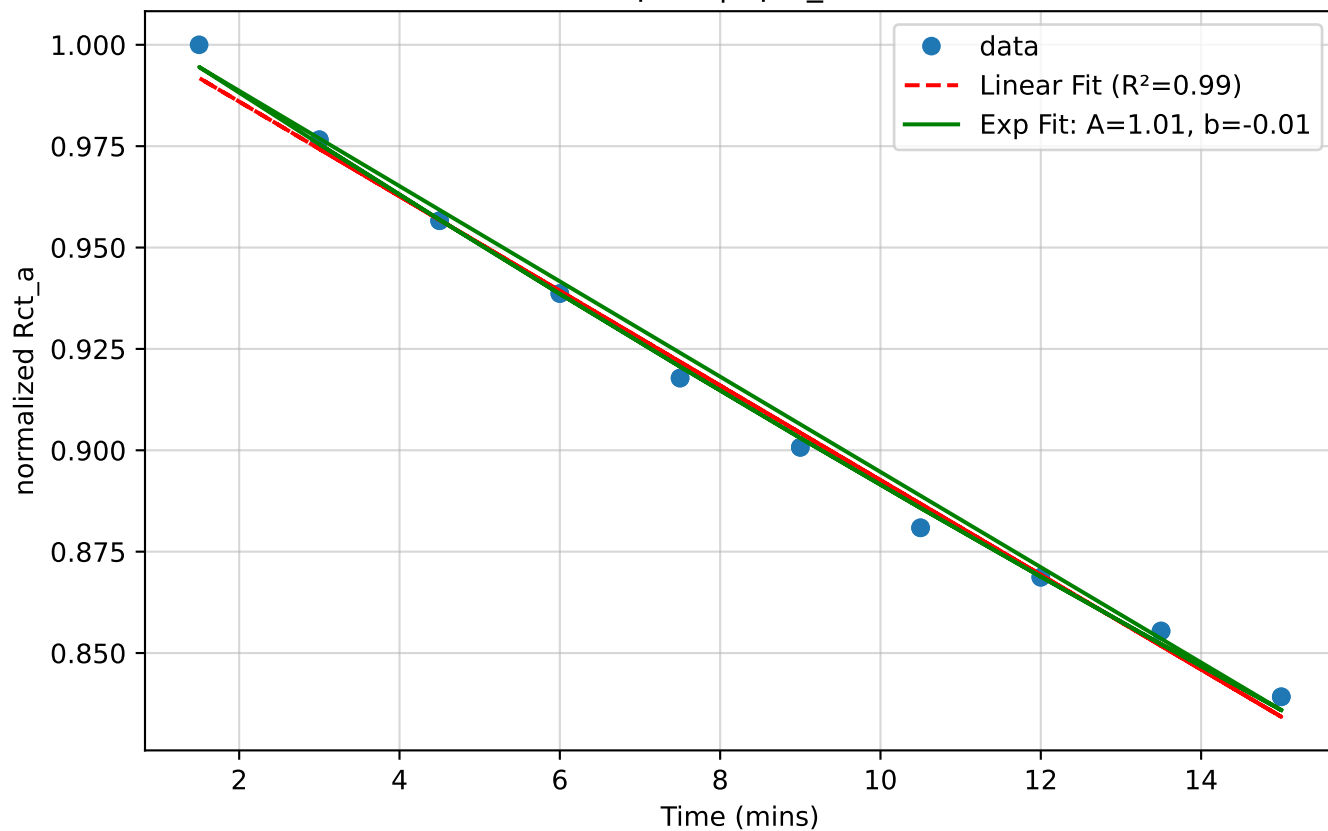
Chip 39 | 0pM_asso
